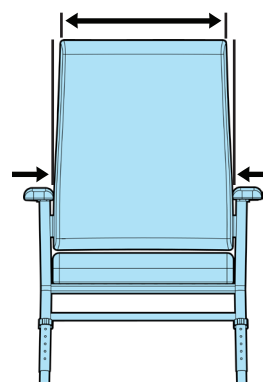
Backrest width 570mm (W - top) 620mm (W - bottom)
